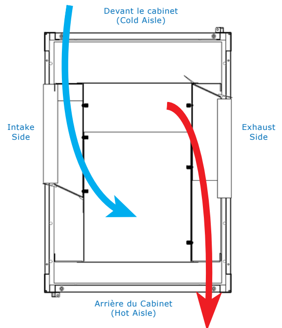
VUE SUPÉRIEURE DE L'ARMOIRE
